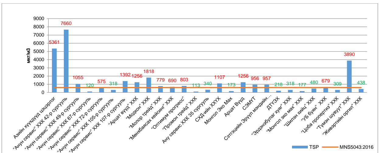
Зураг 20. Усан халаалтын зуухнуудын тоосонцор /TSP/-ын агууламжийн хэмжээ
