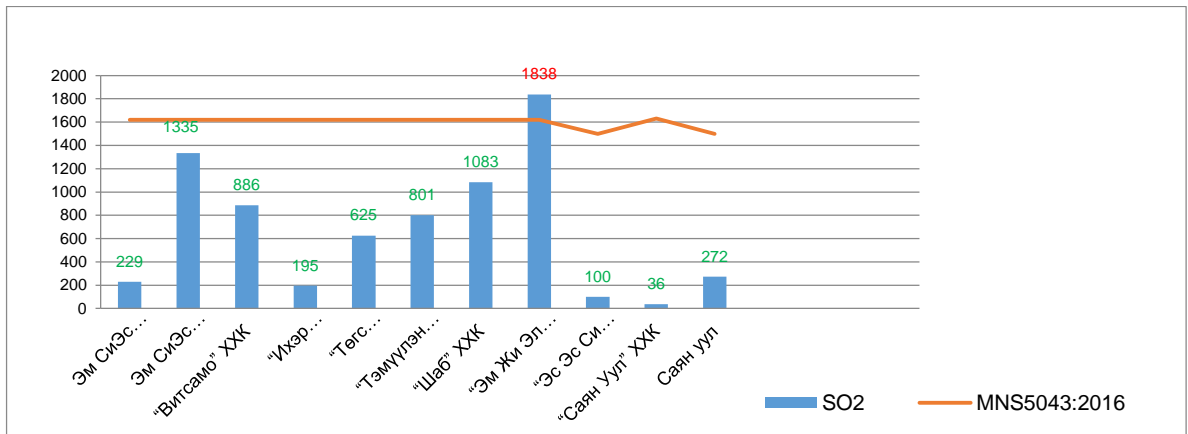
Зураг 18. Уурын зуухнуудын хүхрийн давхар исэл /SO2 /-ийн агууламжийн хэмжээ
