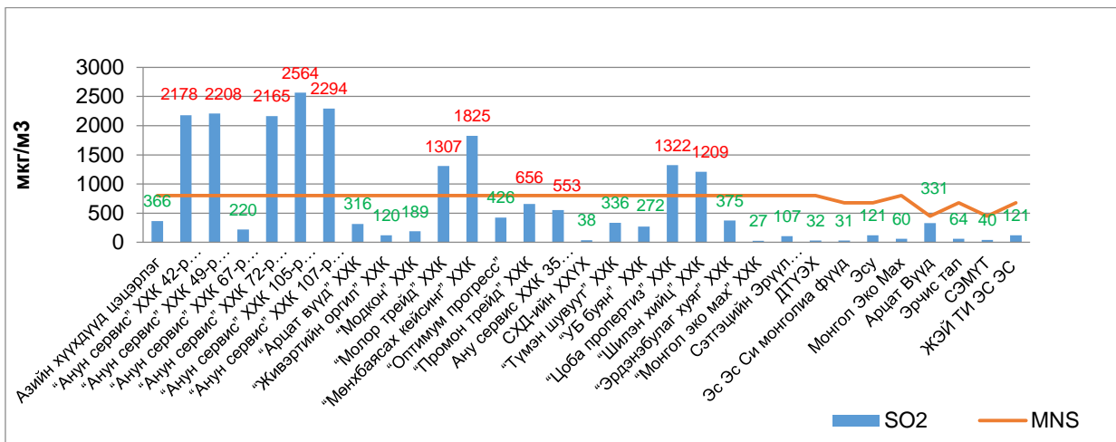
Зураг 21. Усан халаалтын зуухнуудын хүхэрлэг хийн /SO 2 / агууламжийн хэмжээ
