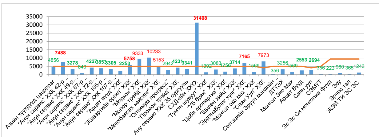
Зураг 22. Усан халаалтын зуухнуудын нүүрстөрөгчийн дутуу ислийн/CO/ агууламжийн хэмжээ
