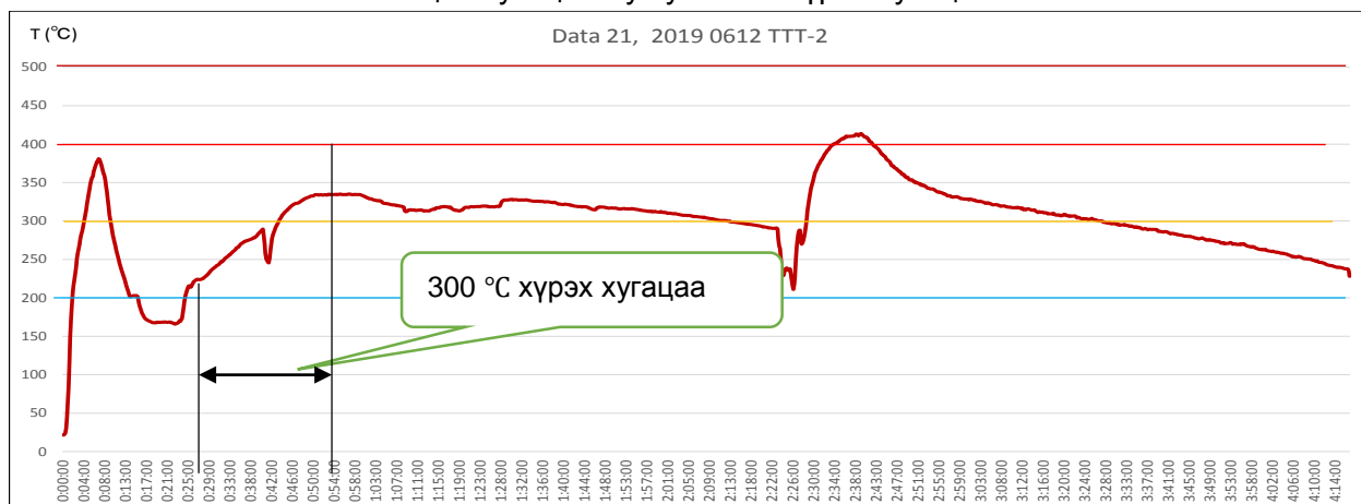
Зураг 23. Таван толгой түлш ХХК-ийн сайжруулсан хатуу түлшний ноцох хугацаа буюу 300°C хүрэх хугацаа
