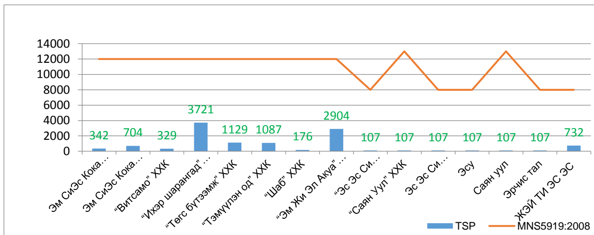
Зураг 17. Уурын зуухнуудын тоосонцор /TSP/- ын агууламжийн хэмжээ
