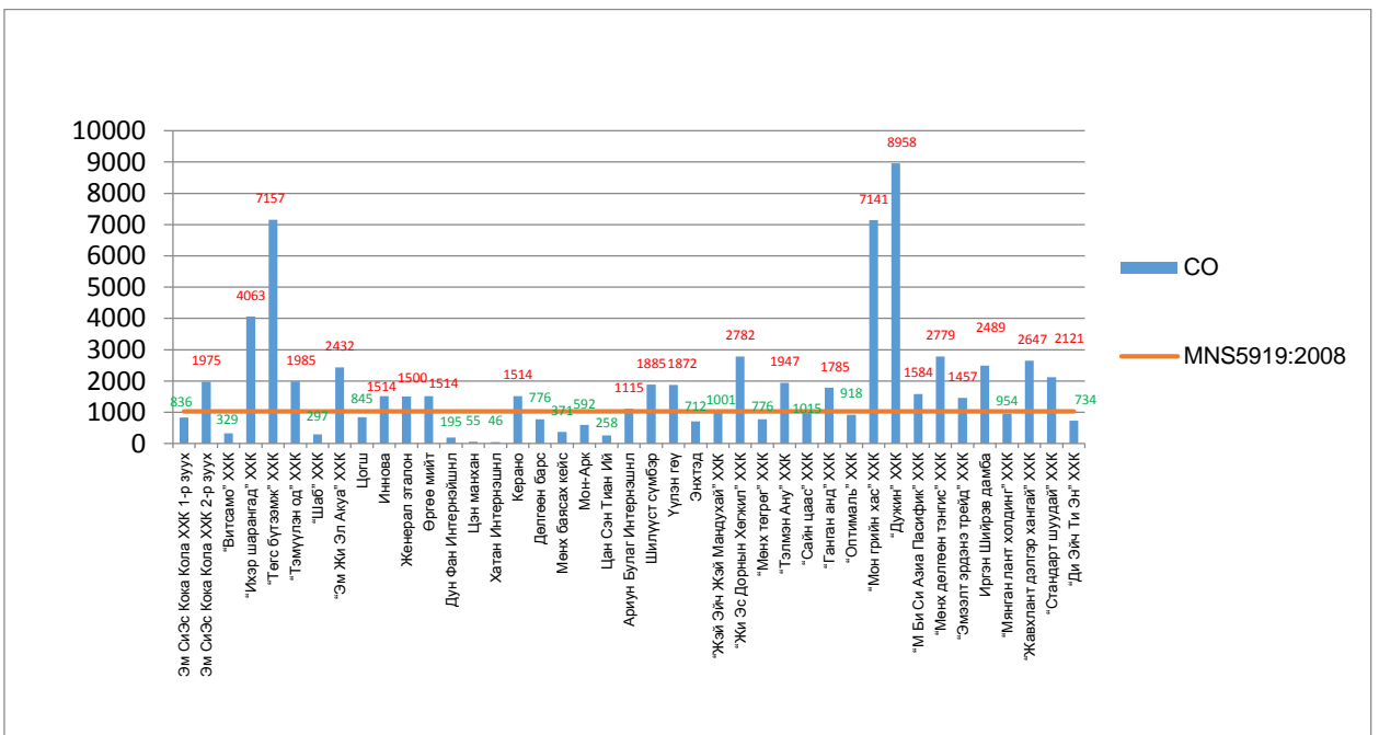
Зураг 30. Уурын зуухнуудын нүүрстөрөгчийн дутуу ислийн /CO/ агууламжийн хэмжээ
